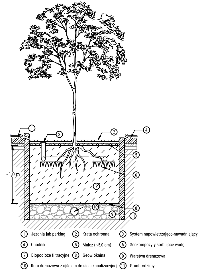
Prosty schemat konstrukcji magazynującej wodę wokół drzewa
