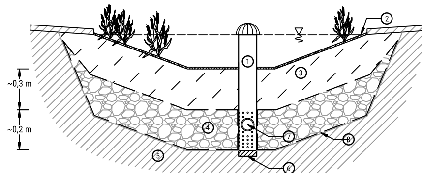
Przekrój ogrodu deszczowego z zastosowaniem warstwy drenażowej do odprowadzania nadmiaru wody
