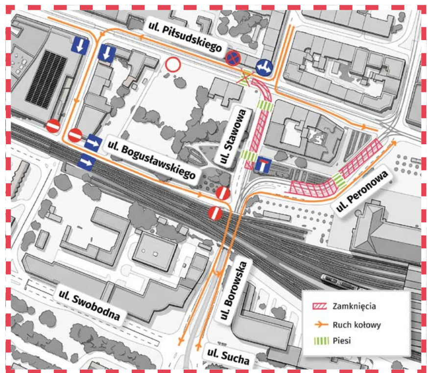
Widok na remontowane odcinki torowiska tramwajowego na skrzyżowaniu przy ul. Stawowej i Peronowej oraz mapa zmian w organizacji ruchu
