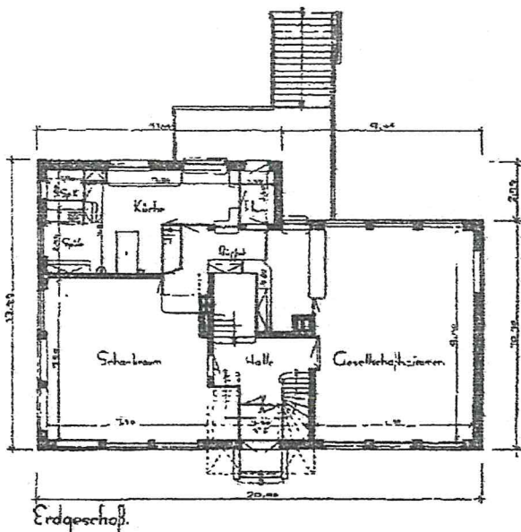
Grundriß: Gesellschaftshaus „Sakrator Wohnhaus“ Toiletten im Keller, von der Erdgesch.-Halle und vom Garten zugänglich. Saal, Toiletten und Gastwirtschaft im Obergeschoß. Im Dachgeschoß 4 Kammern und Bodenraum.
