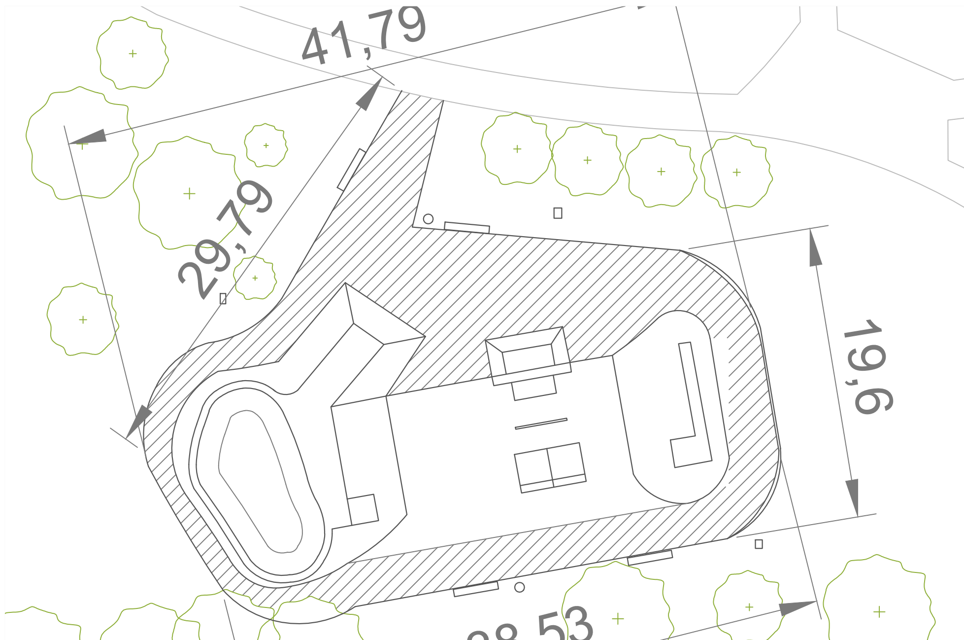
SKATEPARK WIELKA WYSPA RYS. 4 SKATE PARK SKALA 1:250
