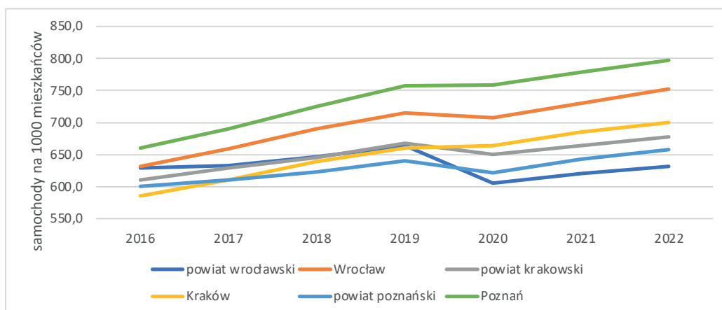
Ryc. 24. Liczba samochodów na 1 tys. mieszkańców w wybranych miastach i powiatach (str. 33)
