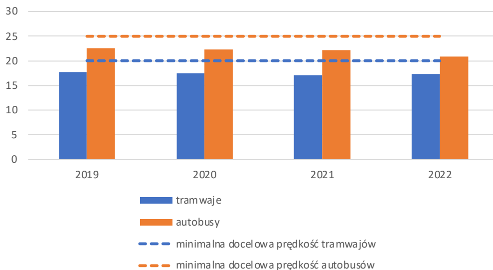
Ryc. 31. Średnia prędkość na liniach tramwajowych i autobusowych we Wrocławiu na tle pożądaney minimalnej prędkości pojazdów.
