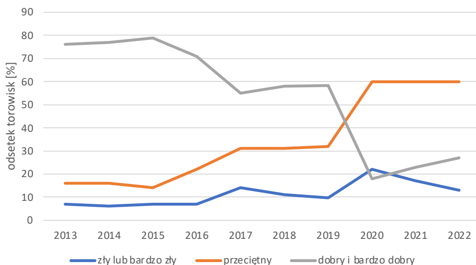
Ryc. 32. Stan techniczny torów tramwajowych we Wrocławiu w latach 2013-2022.
