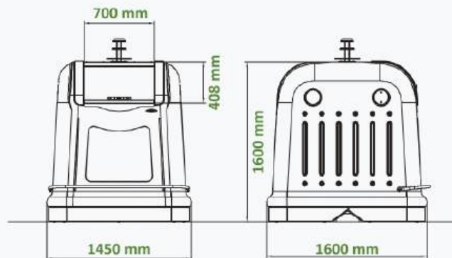
Wymiary pojemnika 3 m 3
